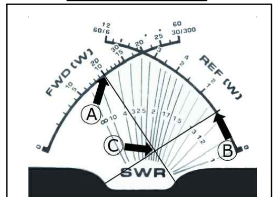
読み取り例 300Wレンジの場合
